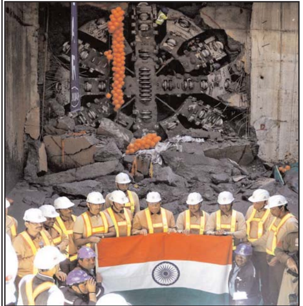
केन्द्रीय मंत्री मनोहर लाल खट्टर नई दिल्ली में दिल्ली मेट्रो के वसंत कुंज टीबीएम परियोजना स्थल पर टीबीएम (टनल बोरिंग मशीन) की सफलता के स्थल का दौरा करते हुए।
